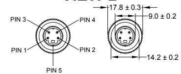
4 PIN MINI DIN MALE MATING FACE
